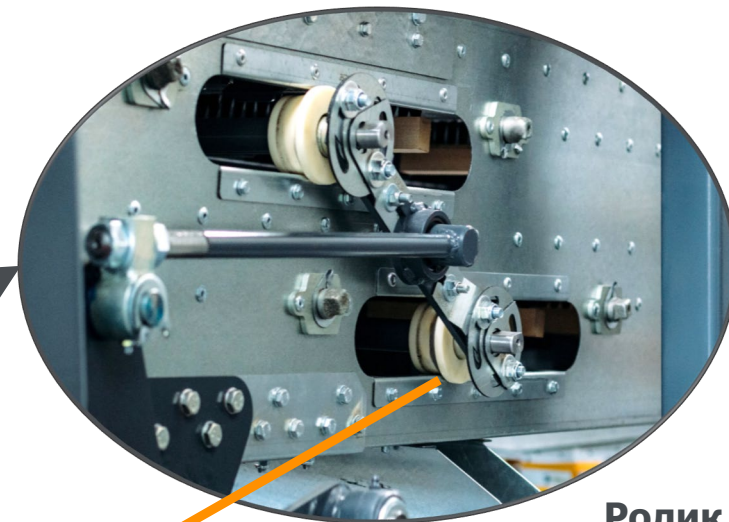
Ролик привода решет
